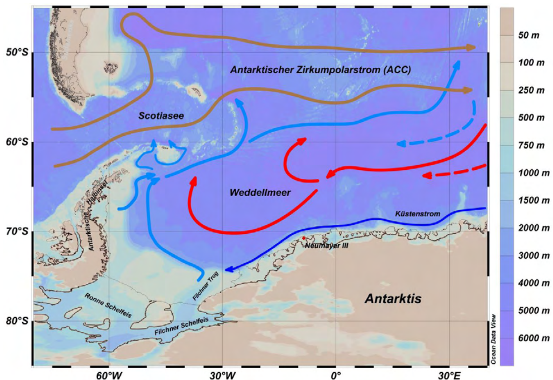
Abbildung II.4.2: Hauptmerkmale der Zirkulation von Wassermassen im Atlantischen Sektor des Südozeans. Braun: Zirkumpolarstrom. Rot: relativ warmes Wasser, das in der Wassersicht um 500 m herum mit dem Weddellwirbel südwestwärts verfrachtet wird. Blau: Kaltwassertransporte; die dünne dunkelblaue Linie zeigt den Antarktischen Küstenstrom, die dickeren hellblauen Linien den Ausstrom frisch gebildeten Bodenwassers. Neumayer III: AWI Forschungsstation (Kap. I.2.1)
